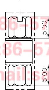
DS TYPE
